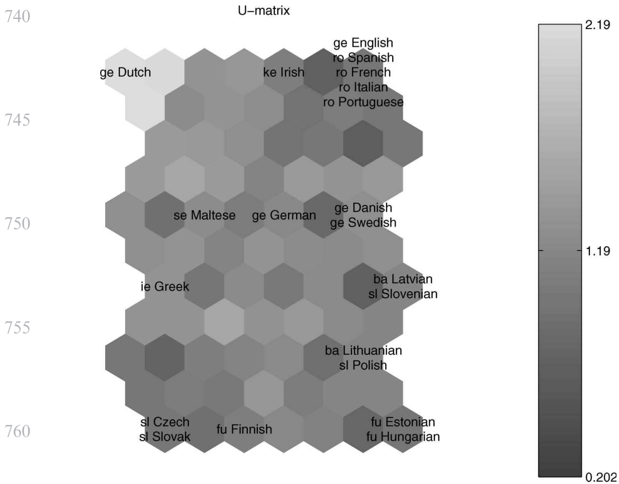
Fig. 7. Official EU languages on the SOM U-matrix.
